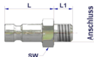
Außengewinde
