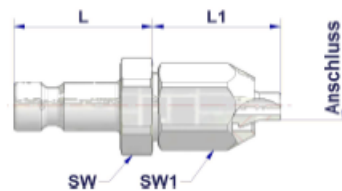
Nippel für Schlauch
