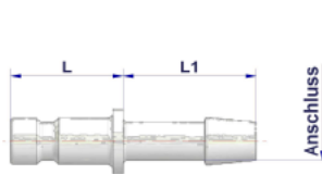
Tülle
