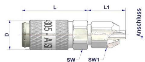
Schlauchanschluss
